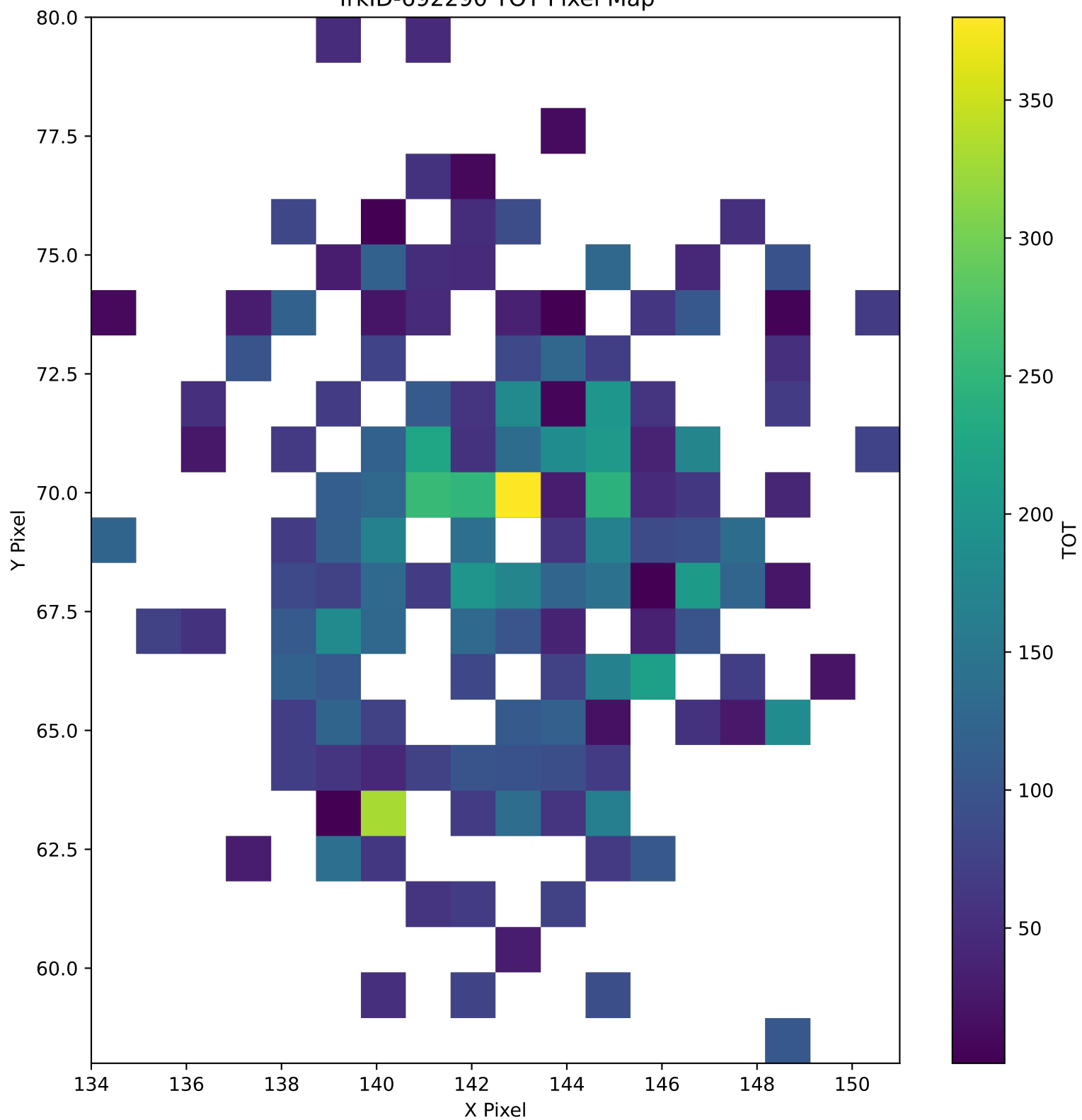
TrkID-692290 TOT Pixel Map
