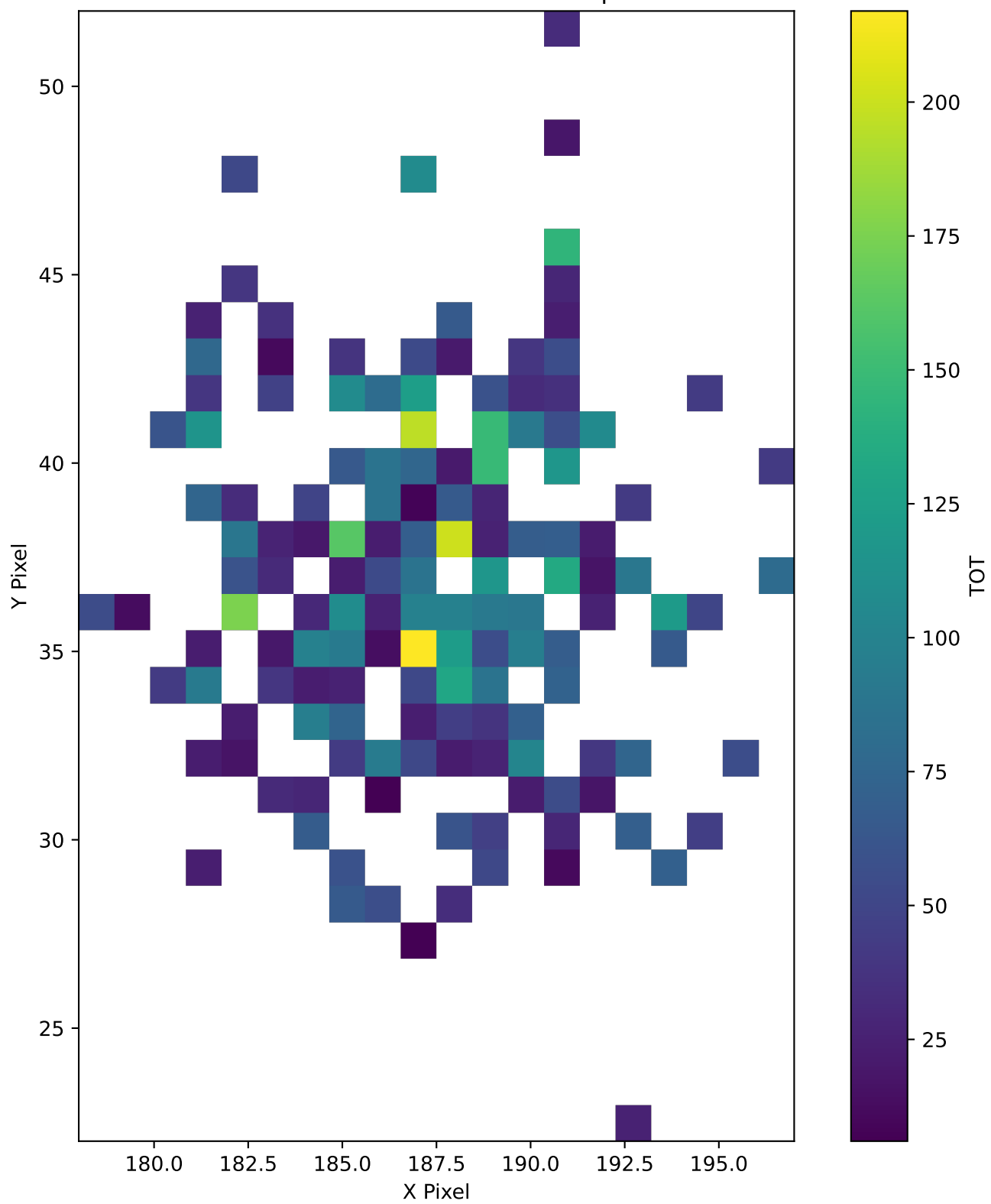
TrkID-1682510 TOT Pixel Map
