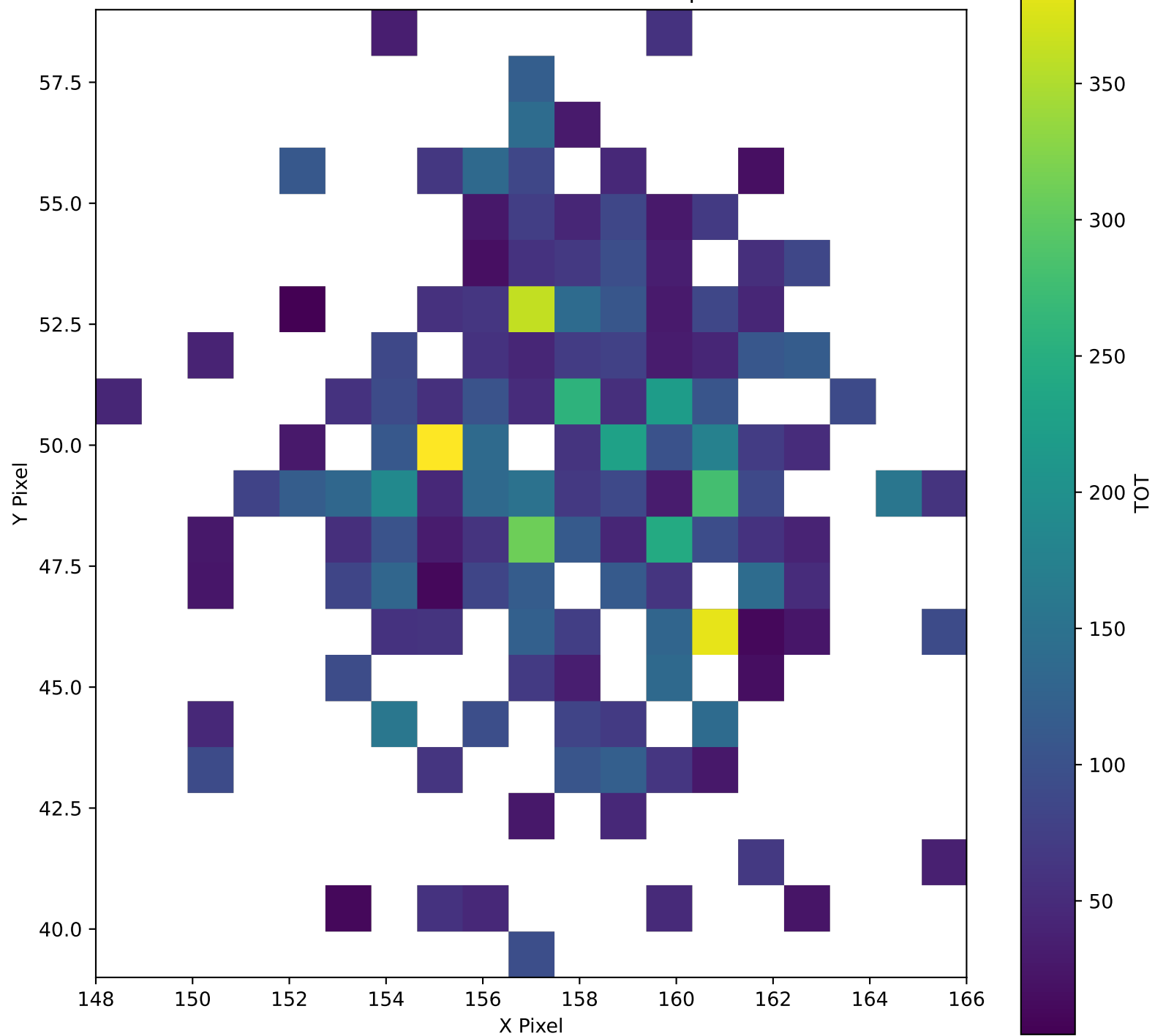
TrkID-2730467 TOT Pixel Map
