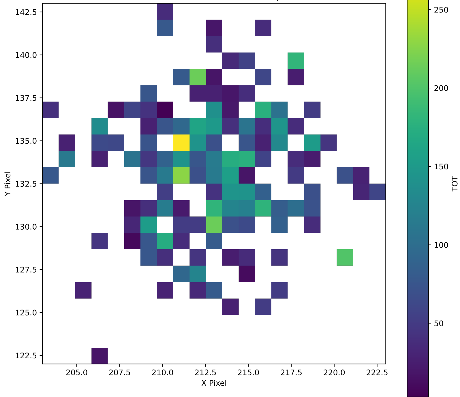
TrkID-3024376 TOT Pixel Map
