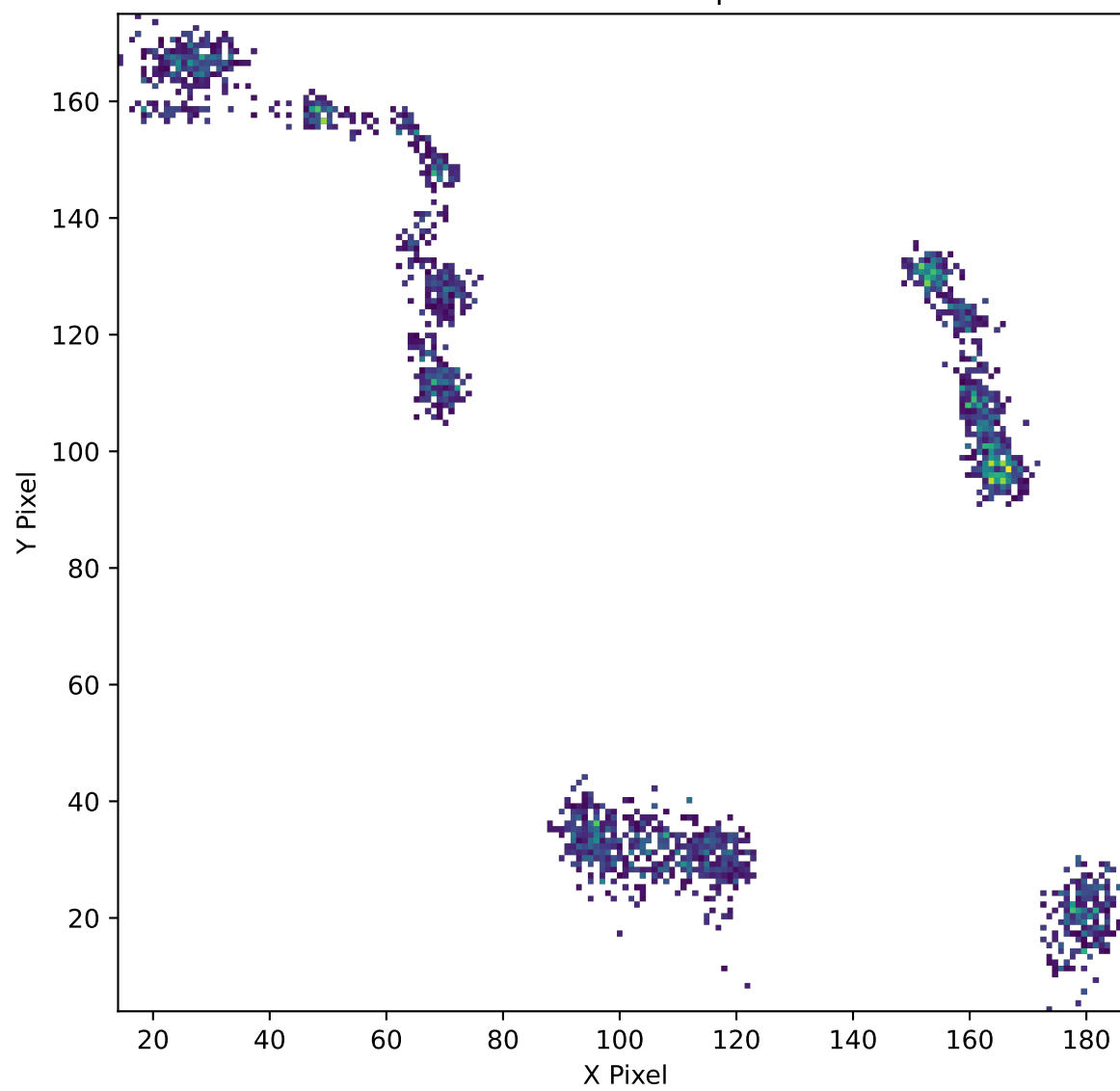
TOT Pixel Map
