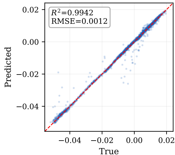
10^{-3} C_l (Roll moment)
