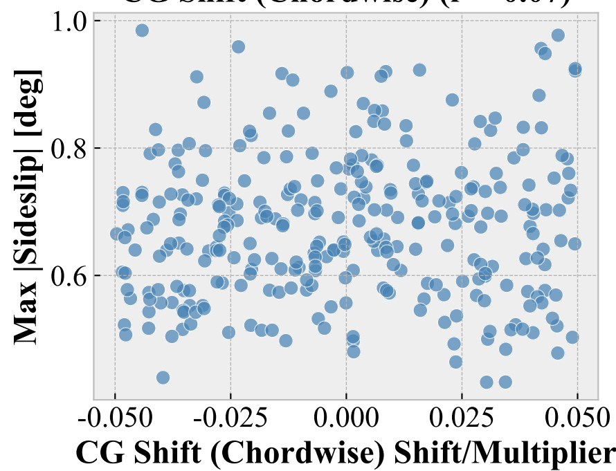
CG Shift (Chordwise) ( r=+0.07 )
