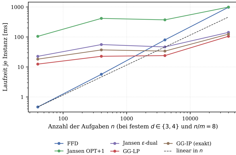
Abbildung 5.10: Laufzeit über n bei festem d \in \{3, 4\} und festem n/m , doppelt logarithmisch. Die gestrichelte Linie wächst linear in n und dient als Bezug.
