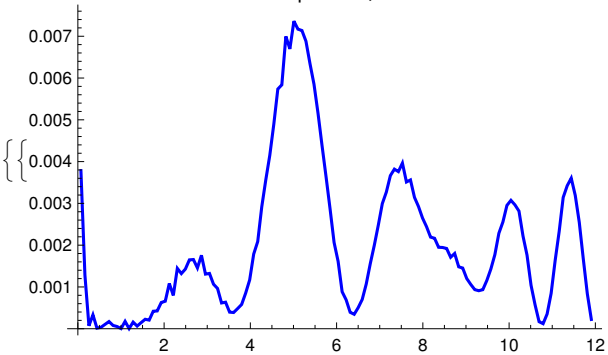
timestep=1000, t=999.
