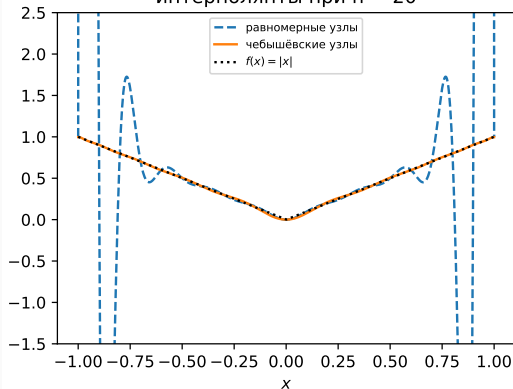
интерполянты при n = 20
