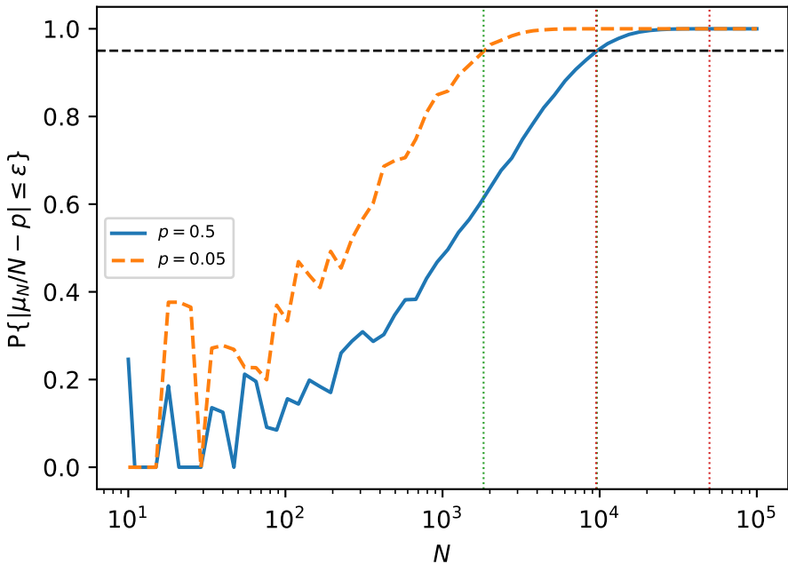
покрытие; пунктир — N по ЦПТ и по Чебышёву
