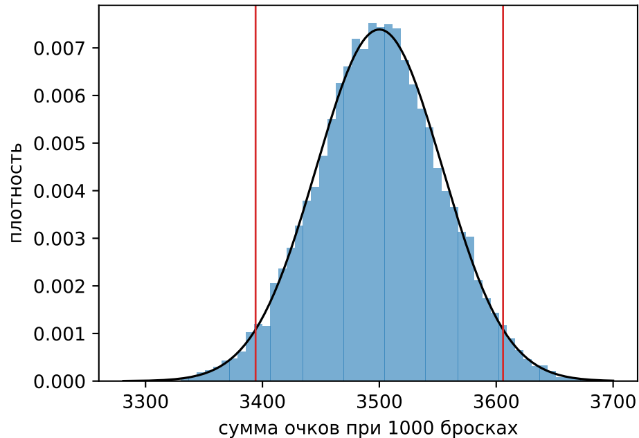
95%-интервал против размаха [1000; 6000]
