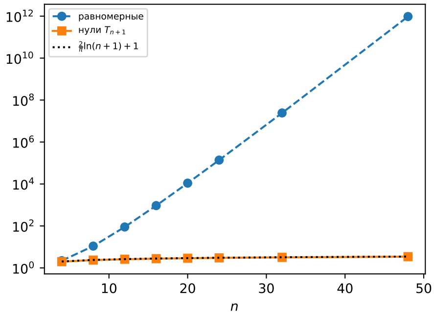
константа Лебега \Lambda_n
