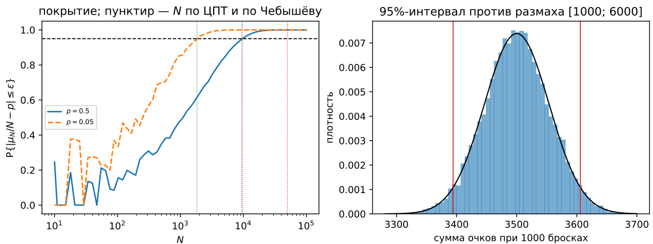
Рис. 4: Слева: точно вычисленная вероятность события \{|\mu_N/N - p| \leq \varepsilon\} как функция N при \varepsilon = 0,01 ; точечные вертикали — объёмы выборки по центральной предельной теореме и по неравенству Чебышёва, горизонталь — заявленный уровень 0,95. Справа: распределение суммы очков при 1000 бросках кости по 20 000 прогонам, нормальная плотность и границы 95 %-интервала. Построено в examples.ipynb , пример 2.
