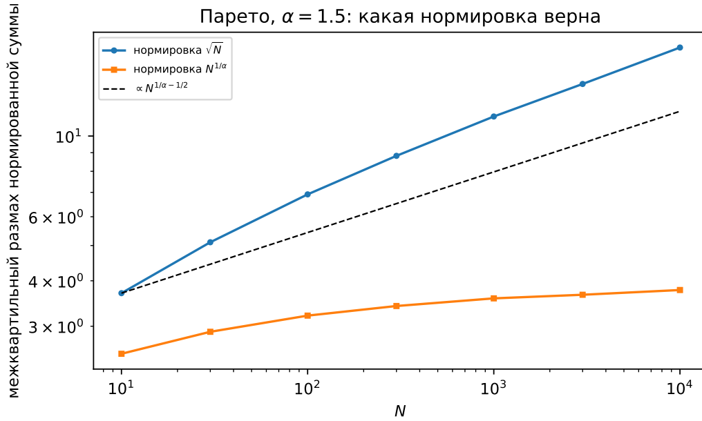
Рис. 3: Закон Парето с \alpha = 1,5 : при нормировке \sqrt{N} межквартильный размах суммы растёт, при нормировке N^{1/\alpha} почти стабилизируется. Наклон первой кривой на последней декаде равен +0,192 при предсказанном 1/\alpha - 1/2 = 1/6 : сходимость к предельному закону при \alpha = 1,5 медленная, и на N \leq 10^4 асимптотика ещё не установилась. Построено в examples.ipynb , пример 4.
