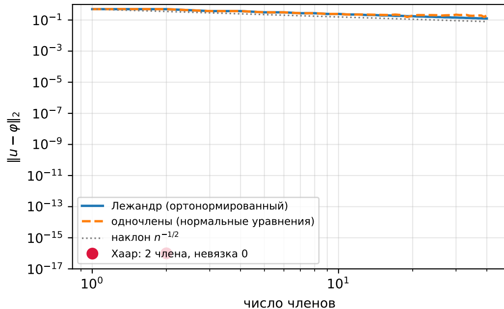
невязка приближения сигнала со скачком
