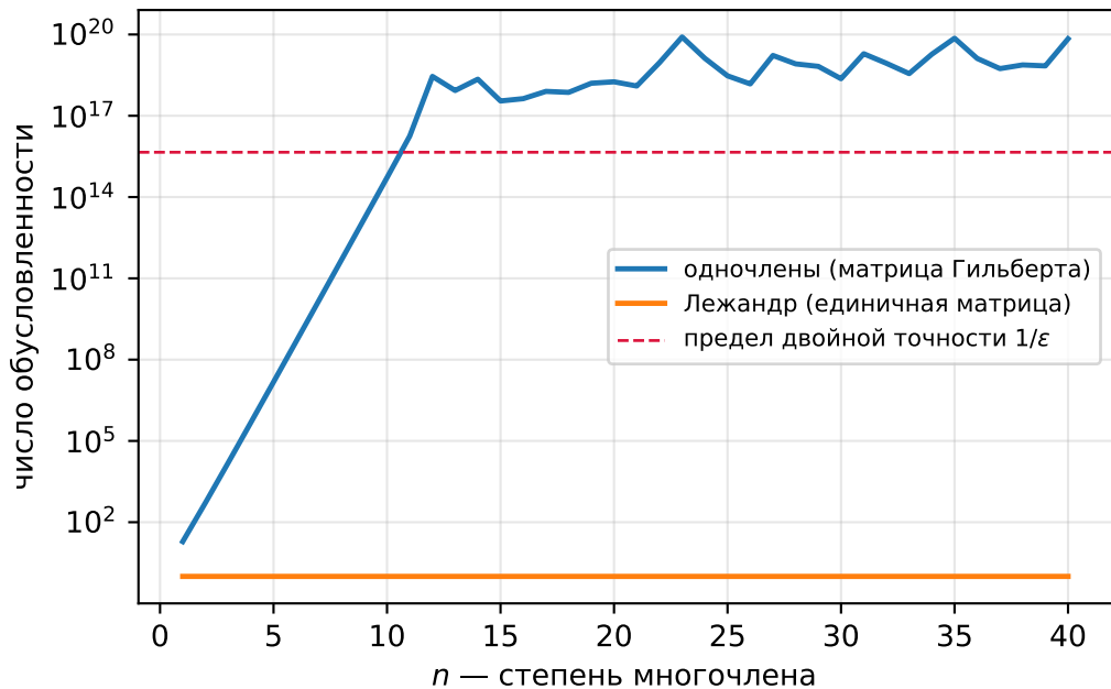
обусловленность матрицы Грама
