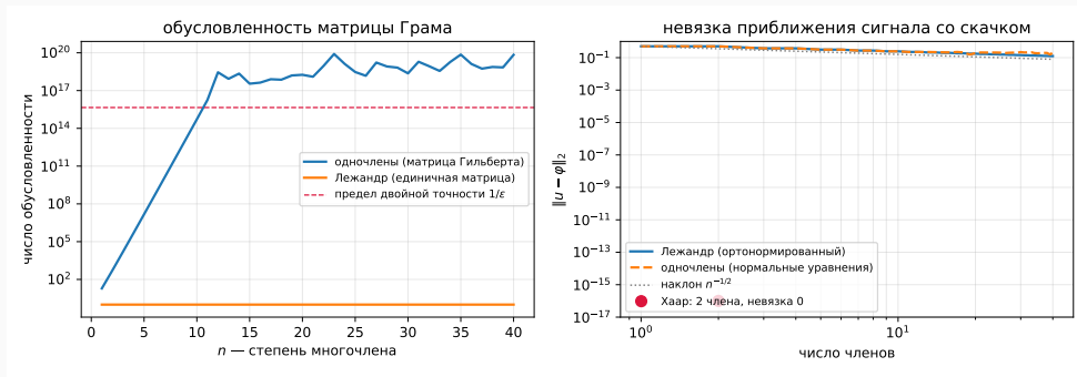
Рис. 4: Слева: обусловленность матрицы Грама одночленов — это матрица Гильберта G_{kl} = 1/(k + l + 1) — при n = 10 равна 5,2 \cdot 10^{14} , у ортонормированного базиса она равна единице. Справа: невязка одна и та же до n = 9 , дальше одночленный путь завышает её — при n = 40 вдвое.
