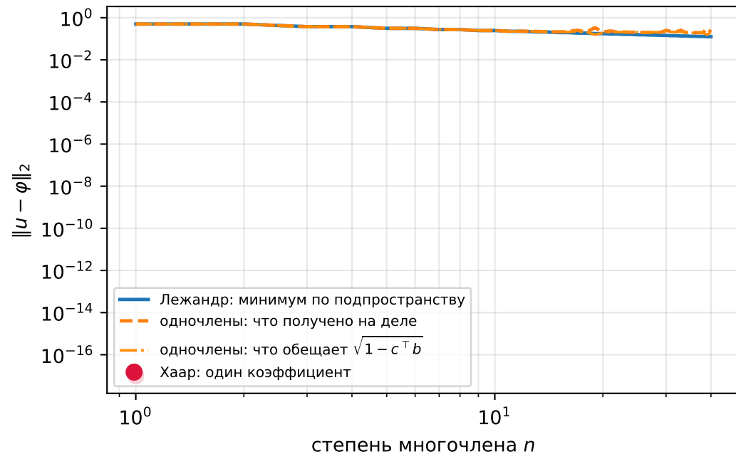
невязка: минимум, достигнутое и обещанное
