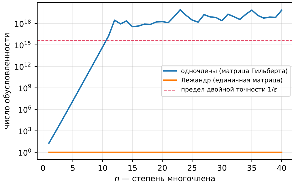
обусловленность матрицы Грама
