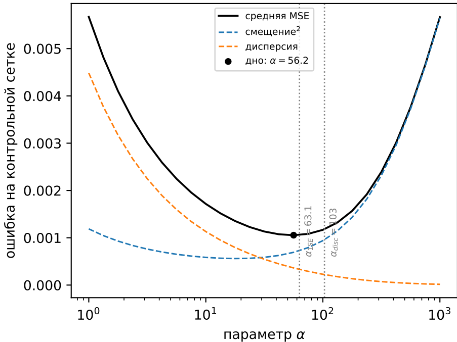
U-образная кривая: смещение растёт, дисперсия падает
