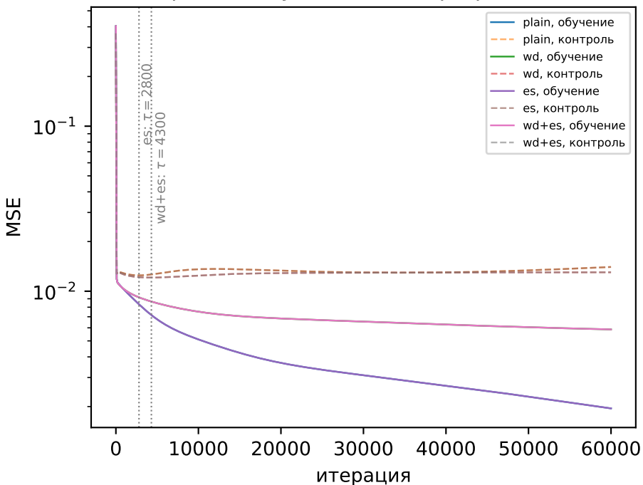
кривые обучения: четыре режима
