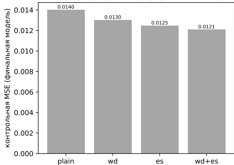
итог: оба регуляризатора улучшают контроль
