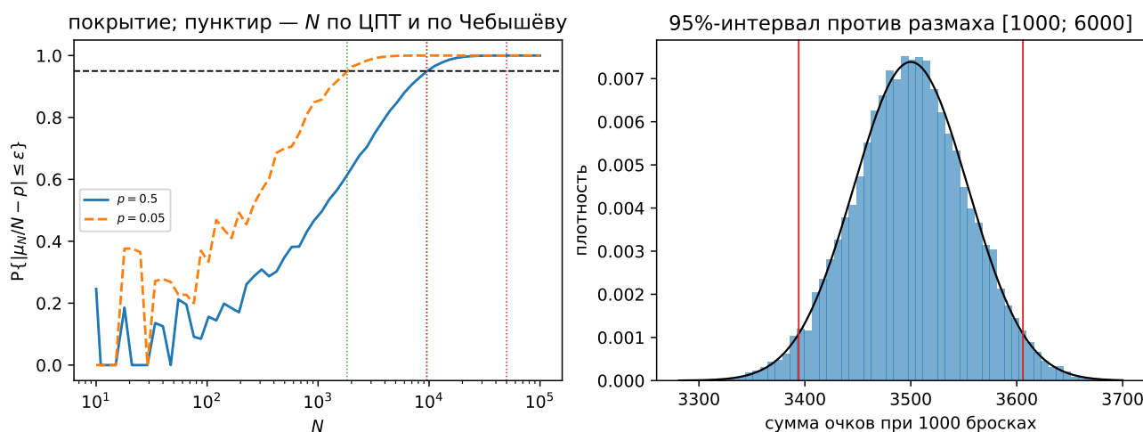
Рис. 3: Слева: точно вычисленная вероятность события \{|\mu_N/N - p| \leq \varepsilon\} как функция N при \varepsilon = 0,01 для p = 0,5 и p = 0,05 ; точечные вертикали — четыре объёма выборки, по два на каждое p : по центральной предельной теореме и по неравенству Чебышёва. Горизонталь — заявленный уровень 0,95. Справа: распределение суммы очков при 1000 бросках кости по 20 000 прогонам, нормальная плотность и границы 95 %-интервала. Построено в examples.ipynb , пример 2.
