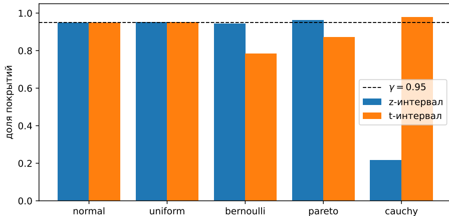
Рис. 1: Доля покрытий z- и t-интервалов при пяти законах шума; пунктир — заявленный уровень \gamma = 0,95 . N = 30, 20\,000 прогонов.
