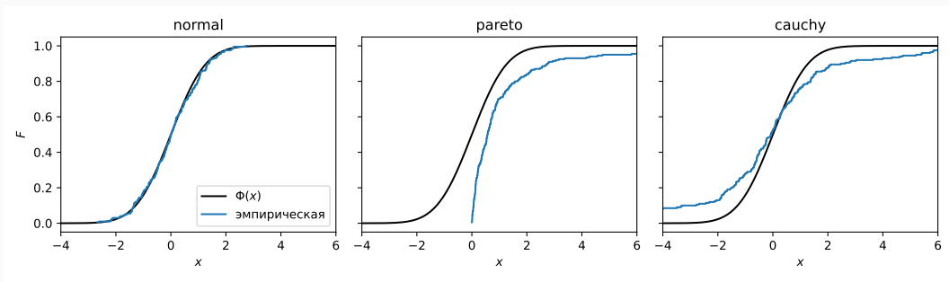
Рис. 3: Эмпирическая функция распределения одной выборки N = 200 против \Phi ; H_0 : выборка из \mathcal{N}(0, 1) .
