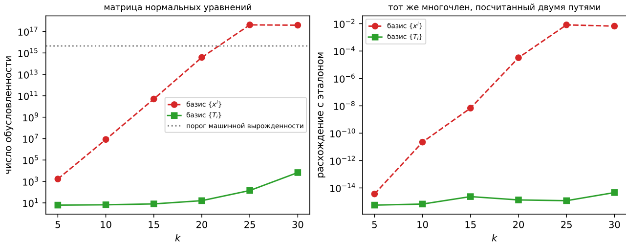
Рис. 4: Слева — число обусловленности матрицы нормальных уравнений в двух базисах; пунктир — порог машинной вырожденности 1/\varepsilon_{\text{маш}} , где \varepsilon_{\text{маш}} — машинная точность, то есть шаг между единицей и следующим представимым числом. Справа — насколько посчитанный многочлен расходится с верным. Построено в examples.ipynb , пример 5.
