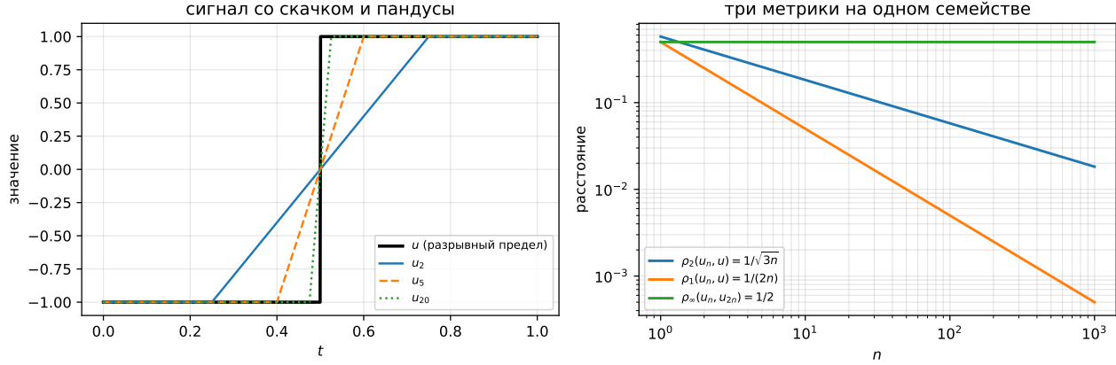
Рис. 1: Сквозной пример в трёх метриках. Слева: разрывный сигнал u и пандусы u_2, u_5, u_{20} , приближающие его. Справа: расстояния от пандуса до u в метриках \rho_1 и \rho_2 убывают как 1/(2n) и 1/\sqrt{3n} , тогда как в равномерной метрике расстояние между u_n и u_{2n} равно 1/2 при любом n и никуда не убывает. Замкнутые формы сверены с точной квадратурой Гаусса; расхождение 10^{-15} . Построено в examples.ipynb , пример 1.
