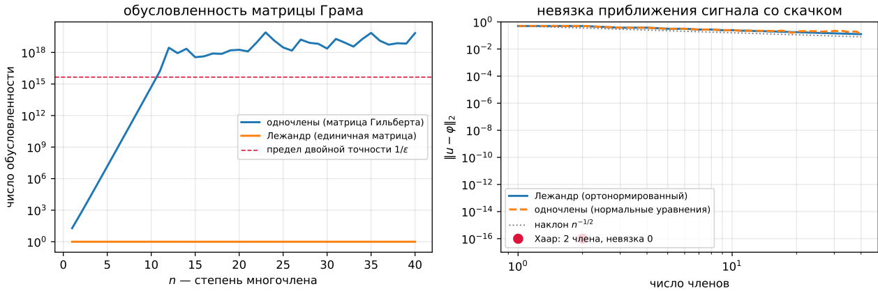
Рис. 4: Цена выбора базиса при одном и том же подпространстве. Слева: обусловленность матрицы Грама одночленов — это матрица Гильберта (32) — растёт экспоненциально и при n = 10 достигает 5,2 \cdot 10^{14} , тогда как у ортонормированного базиса она равна единице. Справа: невязка приближения сигнала со скачком. Оба пути дают одну и ту же невязку до n = 9 , впервые расходятся более чем на 10^{-3} при n = 11 , а дальше одночленный путь завышает её — при n = 40 вдвое. Система Хаара даёт нулевую невязку двумя членами. Построено в examples.ipynb , пример 3.
