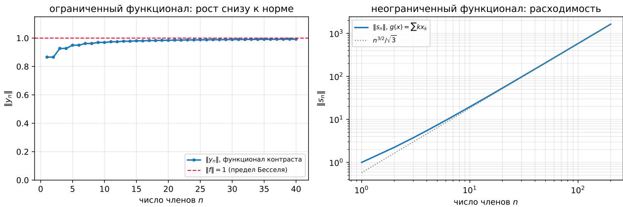
Рис. 3: Конструктивное доказательство как проверка существования представителя. Слева: частичные нормы \|y_n\| для функционала контраста растут монотонно и снизу к \|f\| = 1 — это неравенство Бесселя (20) вместе с оценкой (27). Справа: для неограниченного функционала g(x) = \sum_k kx_k те же частичные нормы уходят на бесконечность с измеренным наклоном 1,48 на диапазоне n от 5 до 200, подходящим к предельному 3/2 снизу. Построено в examples.ipynb , пример 4.
