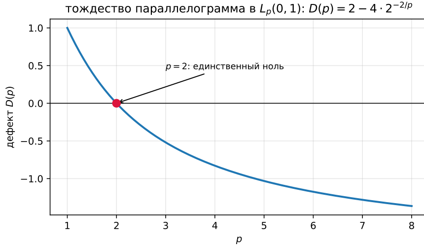
Рис. 2: Дефект тождества параллелограмма в L_p(0, 1) на паре индикаторов половин отрезка: D(p) = 2 - 4 \cdot 2^{-2/p} . Ноль достигается ровно при p = 2 — единственной норме семейства, порождённой скалярным произведением. Построено в examples.ipynb , пример 2.
