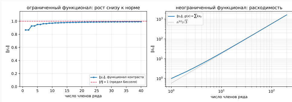
Рис. 3: Слева: частичные нормы представителя контраста растут монотонно и снизу к \|f\| = 1 — неравенство Бесселя в действии. Справа: у неограниченного функционала те же частичные нормы расходятся, измеренный наклон 1,48 на диапазоне от 5 до 200 подходит к предельному 3/2 снизу.
