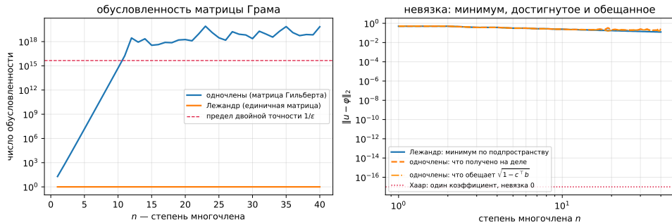
Рис. 4: Слева: обусловленность матрицы Грама одночленов — это матрица Гильберта G_{kl} = 1/(k + l + 1) — при n = 10 равна 5,2 \cdot 10^{14} , у ортонормированного базиса она равна единице. Справа: минимум по подпространству, фактически полученная невязка и то, что обещает тождество. Первые две совпадают до n = 11 ; при n = 18 завышение 11,0 %, при n = 40 — в 1,64 раза. Третья при n = 11, 12, 19 уходит ниже минимума — чего не может дать ни один элемент подпространства.
