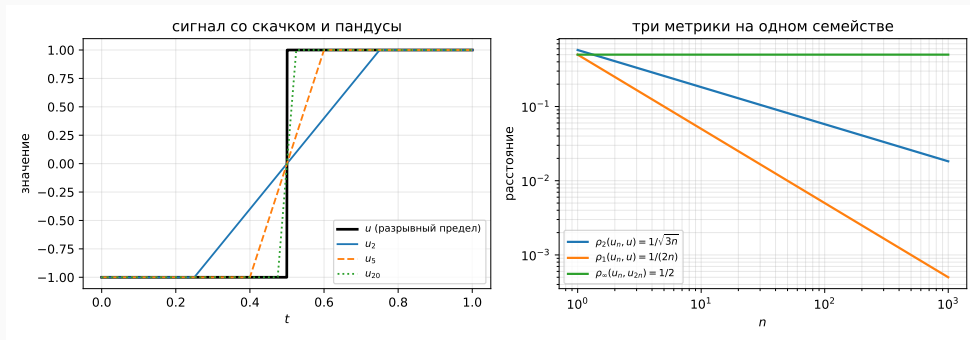
Рис. 1: Слева: сигнал u и пандусы. Справа: в метриках \rho_1 и \rho_2 расстояние до u убывает как 1/(2n) и 1/\sqrt{3n} , а в равномерной метрике расстояние между u_n и u_{2n} равно 1/2 при любом n .
