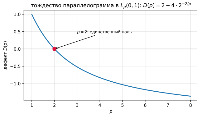
Рис. 2: Дефект тождества параллелограмма D(p) = 2 - 4 \cdot 2^{-2/p} . Единственный ноль — при p = 2 : только среднеквадратичная норма порождена скалярным произведением, и только к ней применима теорема о проекции.
