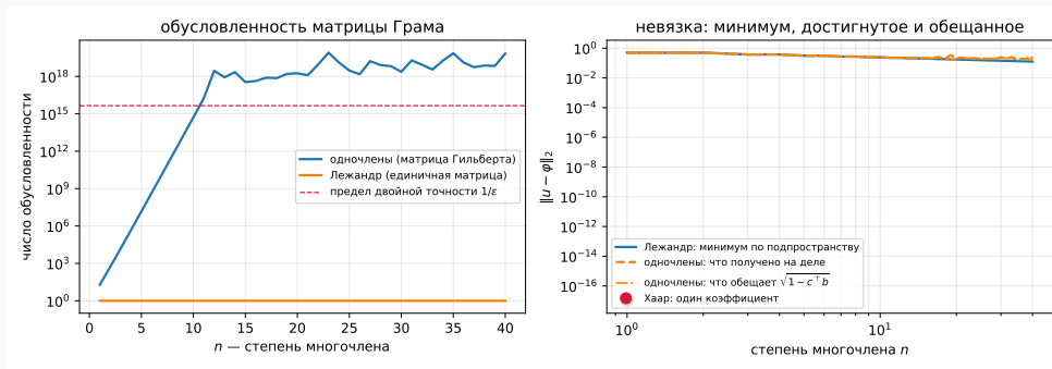
Рис. 4: Слева: обусловленность матрицы Грама одночленов — это матрица Гильберта G_{kl} = 1/(k + l + 1) — при n = 10 равна 5,2 \cdot 10^{14} , у ортонормированного базиса она равна единице. Справа: минимум по подпространству, фактически полученная невязка и то, что обещает тождество. Первые две совпадают до n = 11 ; при n = 18 завышение 11,0 %, при n = 40 — в 1,64 раза.
