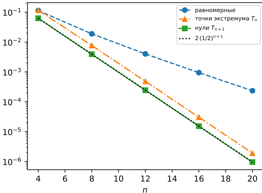
\|\omega_{n+1}\|_{C[-1,1]}
