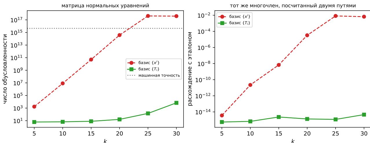
Рис. 5: Слева — число обусловленности матрицы нормальных уравнений в двух базисах на n = 60 равномерных узлах; пунктир — машинная точность 1/\varepsilon_{\text{маш}} . Справа — насколько посчитанный многочлен расходится с верным. Подпространство одно и то же, разница целиком вычислительная. Построено в examples.ipynb , пример 5.
