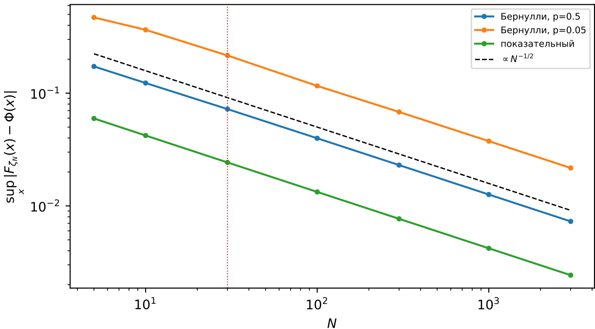
скорость сходимости в ЦПТ; пунктир — граница N = 30
