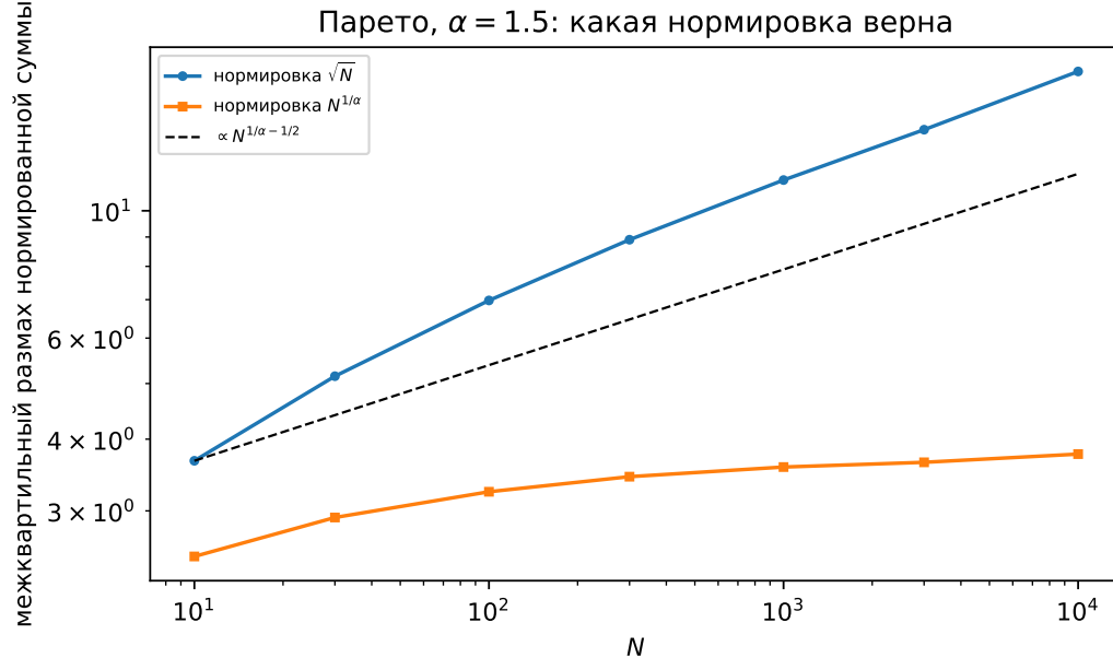
Рис. 3: Закон Парето с \alpha = 1,5 : при нормировке \sqrt{N} межквартильный размах суммы растёт, при нормировке N^{1/\alpha} почти стабилизируется. Разность наклонов в логарифмических осях равна 1/\alpha - 1/2 = 1/6 с точностью до шестого знака — показатель нормировки определён однозначно и не равен 1/2 . Построено в examples.ipynb , пример 4.
