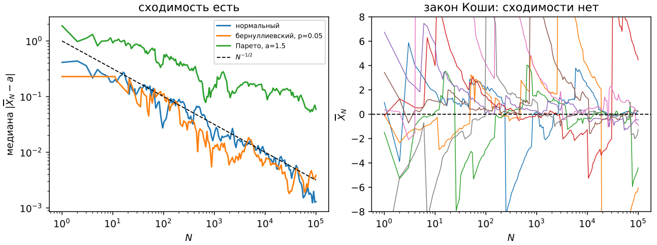
Рис. 1: Слева: медиана уклонения |\bar{X}_N - a| по восьми прогонам для трёх законов с конечным средним; пунктир — эталон N^{-1/2} . Закон Парето с \alpha = 1,5 сходится, но медленнее и ступенями: каждая ступень — одно большое наблюдение. Справа: восемь траекторий \bar{X}_N для закона Коши; сходимости нет ни в одном смысле, и разброс не сужается. Построено в examples.ipynb , пример 1.
