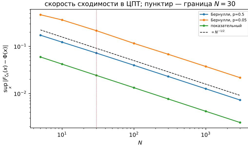
Рис. 2: Скорость сходимости в центральной предельной теореме: точно вычисленное отклонение \sup_x |F_{\zeta_N}(x) - \Phi(x)| для трёх законов (у первых двух сумма биномиальна, у третьего — гамма, поэтому моделирование не нужно). Наклон у всех трёх равен -1/2 , а различаются они множителем; вертикальный пунктир — граница N = 30 , на которой для бернуллиевского закона с p = 0,05 отклонение всё ещё равно 0,216. Построено в examples.ipynb , пример 3.
