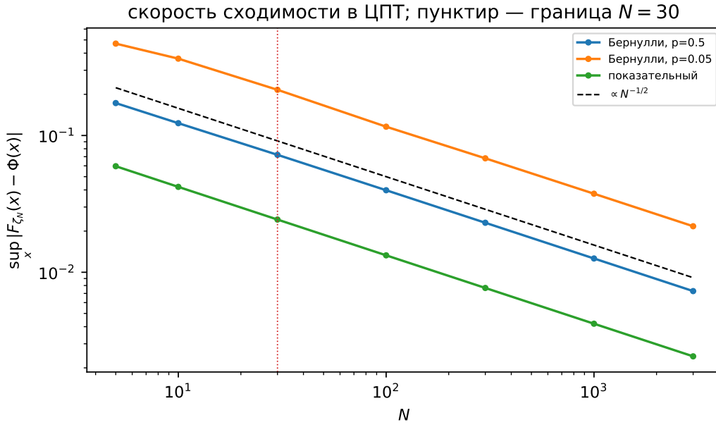
Рис. 4: Скорость сходимости в центральной предельной теореме: уклонение \Delta_N , посчитанное без моделирования (у первых двух сумма биномиальная, у третьего — гамма, поэтому моделирование не нужно). Наклон у всех трёх равен -1/2 , а различаются они множителем; вертикальный пунктир — граница N = 30 , на которой для бернуллиевского закона с p = 0,05 уклонение всё ещё равно 0,216 . Построено в examples.ipynb , пример 3.
