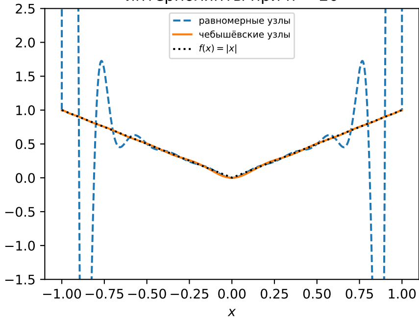
интерполянты при n = 20
