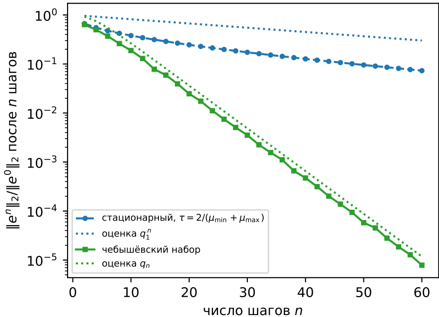
сходимость, \kappa = 100
