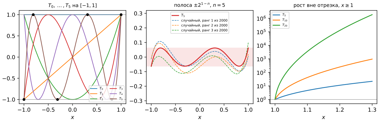
Рис. 1: Слева — T_0, \dots, T_5 на [-1, 1] ; точками отмечены n+1 точка чередования T_5 из (5), в них T_5 = \pm 1 . В середине — приведённый \tilde{T}_5 и три самых удачных из двух тысяч случайных приведённых многочленов пятой степени: полоса \pm 2^{-4} не перекрыта ни одним из них (теорема 4.3). Справа — рост T_n правее единицы в логарифмическом масштабе (теорема 3.4): T_{20}(1,1) = 3562,5 . Построено в examples.ipynb , пример 1.
