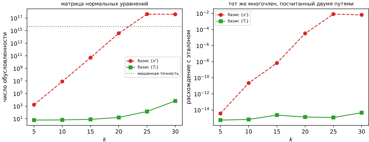
Рис. 4: Слева — число обусловленности матрицы нормальных уравнений в двух базисах на n = 60 равномерных узлах; пунктир — машинная точность 1/\varepsilon_{\text{маш}} . Справа — насколько посчитанный многочлен расходится с верным. Подпространство одно и то же, разница целиком вычислительная. Построено в examples.ipynb, пример 5.
