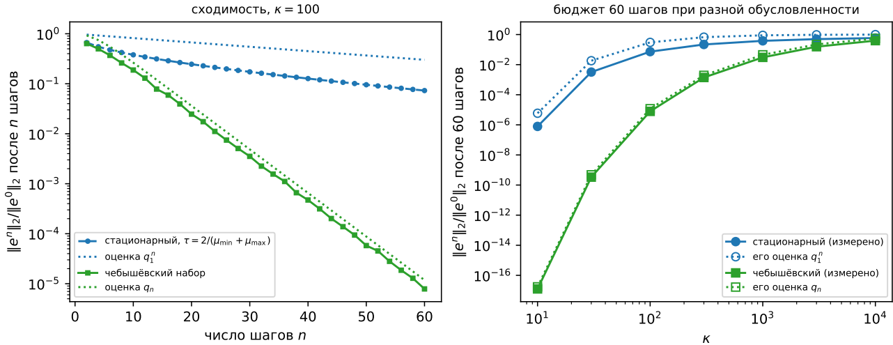
Рис. 3: Слева — погрешность после n шагов при \kappa = 100 (набор параметров пересчитан для каждого n ). Справа — что даёт бюджет в 60 шагов при разной обусловленности: сплошные линии измерены, пунктир — оценки q_n и q_1^n . Выигрыш падает с ростом \kappa , потому что шестидесяти шагов для большой обусловленности уже мало. Построено в examples.ipynb , пример 4.
