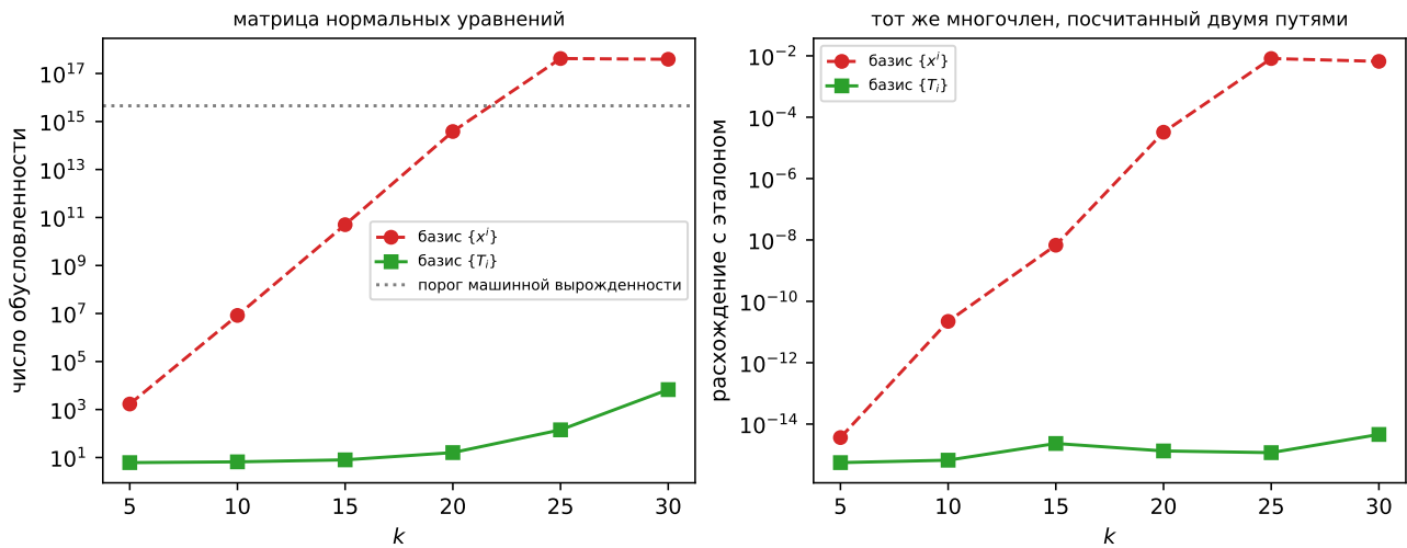
Рис. 4: Слева — число обусловленности матрицы нормальных уравнений в двух базисах; пунктир — порог машинной вырожденности 1/\varepsilon_{\text{маш}} . Справа — насколько посчитанный многочлен расходится с верным. Построено в examples.ipynb , пример 5.
