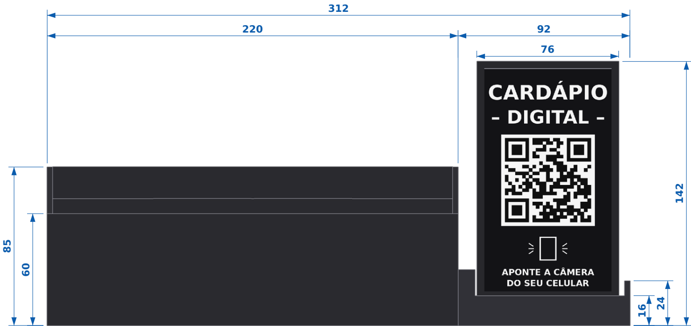
VISTA FRONTAL ESC 1:2
