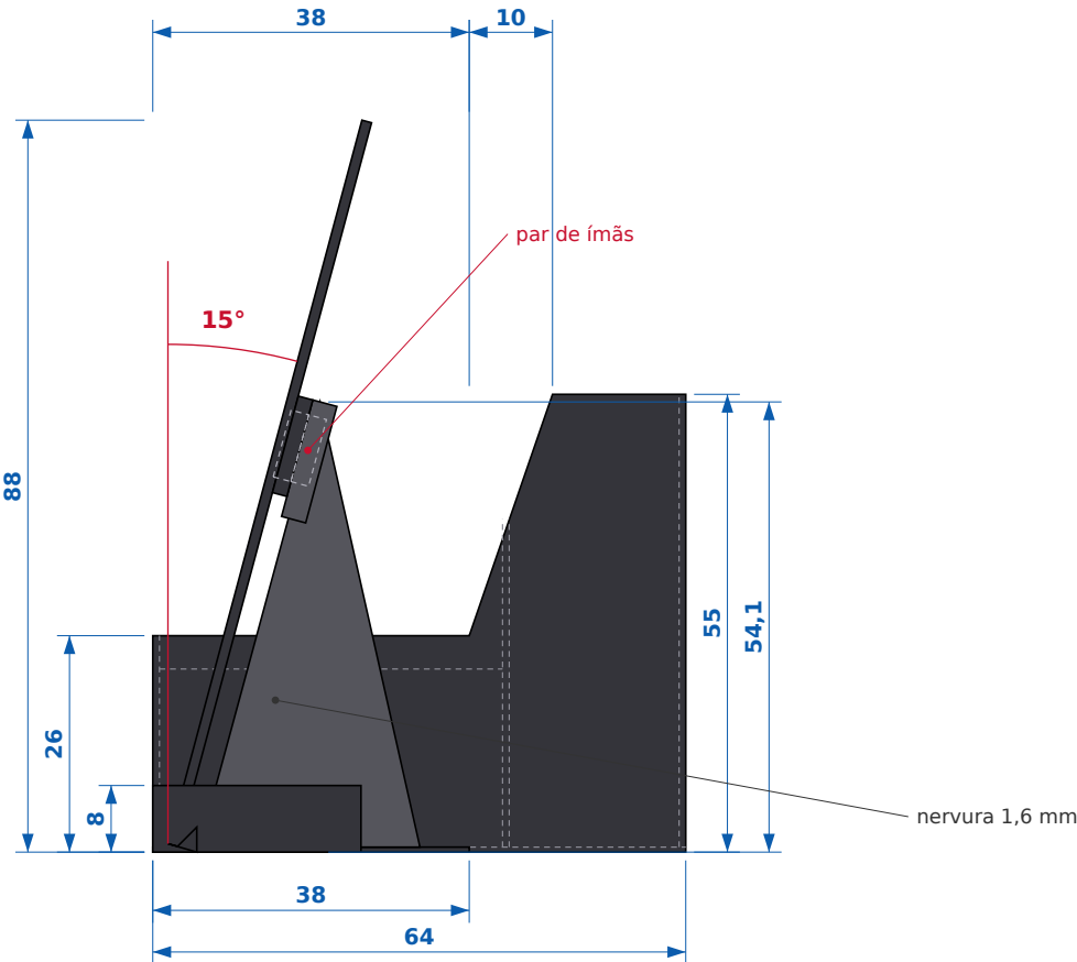
VISTA LATERAL DIREITA ESC 1:1
