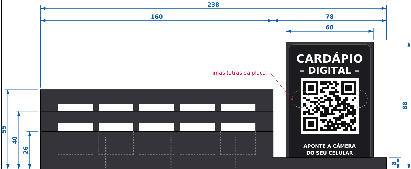
VISTA FRONTAL ESC 1:1,5
