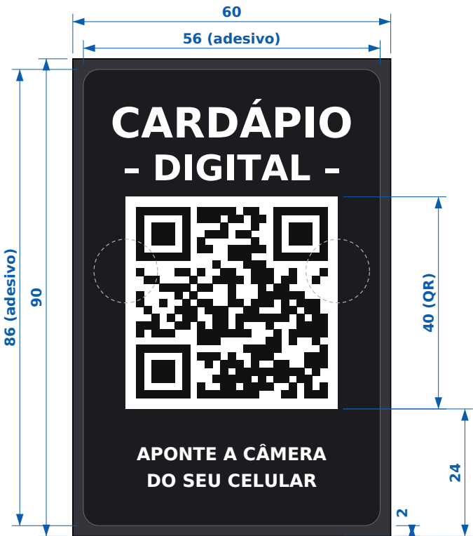
PLACA - FRENTE ESC 1:1 (com adesivo)
