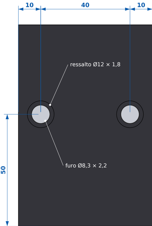
PLACA - VERSO ESC 1:1
