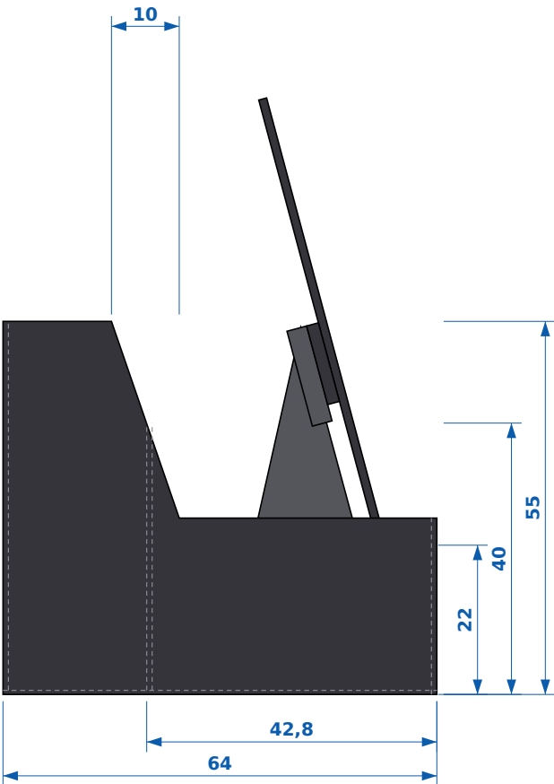
VISTA LATERAL ESQUERDA ESC 1:1
