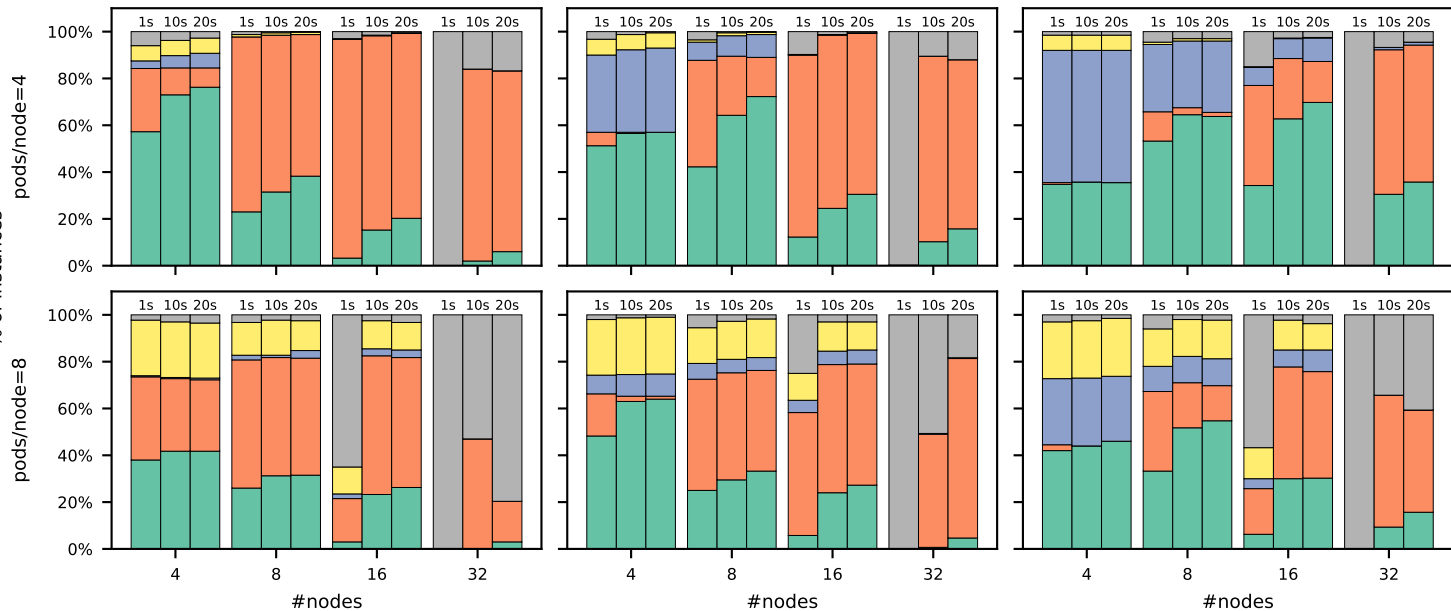
#priorities=1
