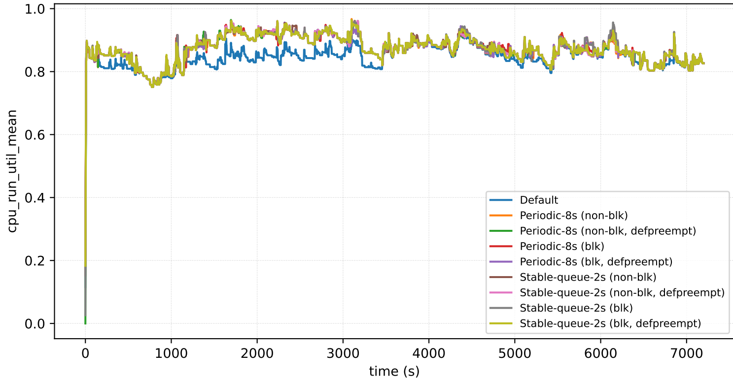
nodes=16_prio=1_arrival=16s: cpu_run_util_mean
