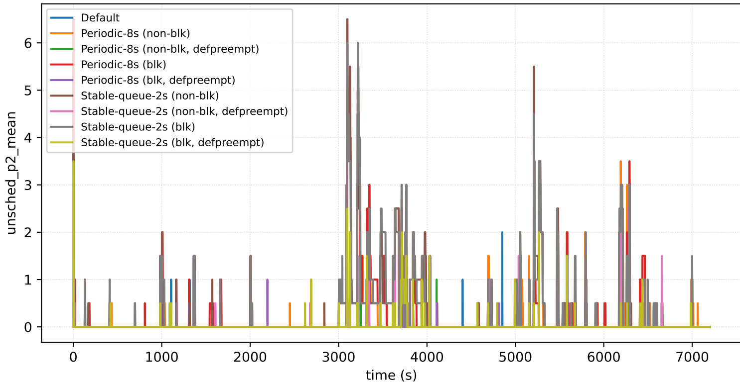
nodes=16_prio=4_arrival=16s: unsched_p2_mean
