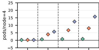
#priorities=1
