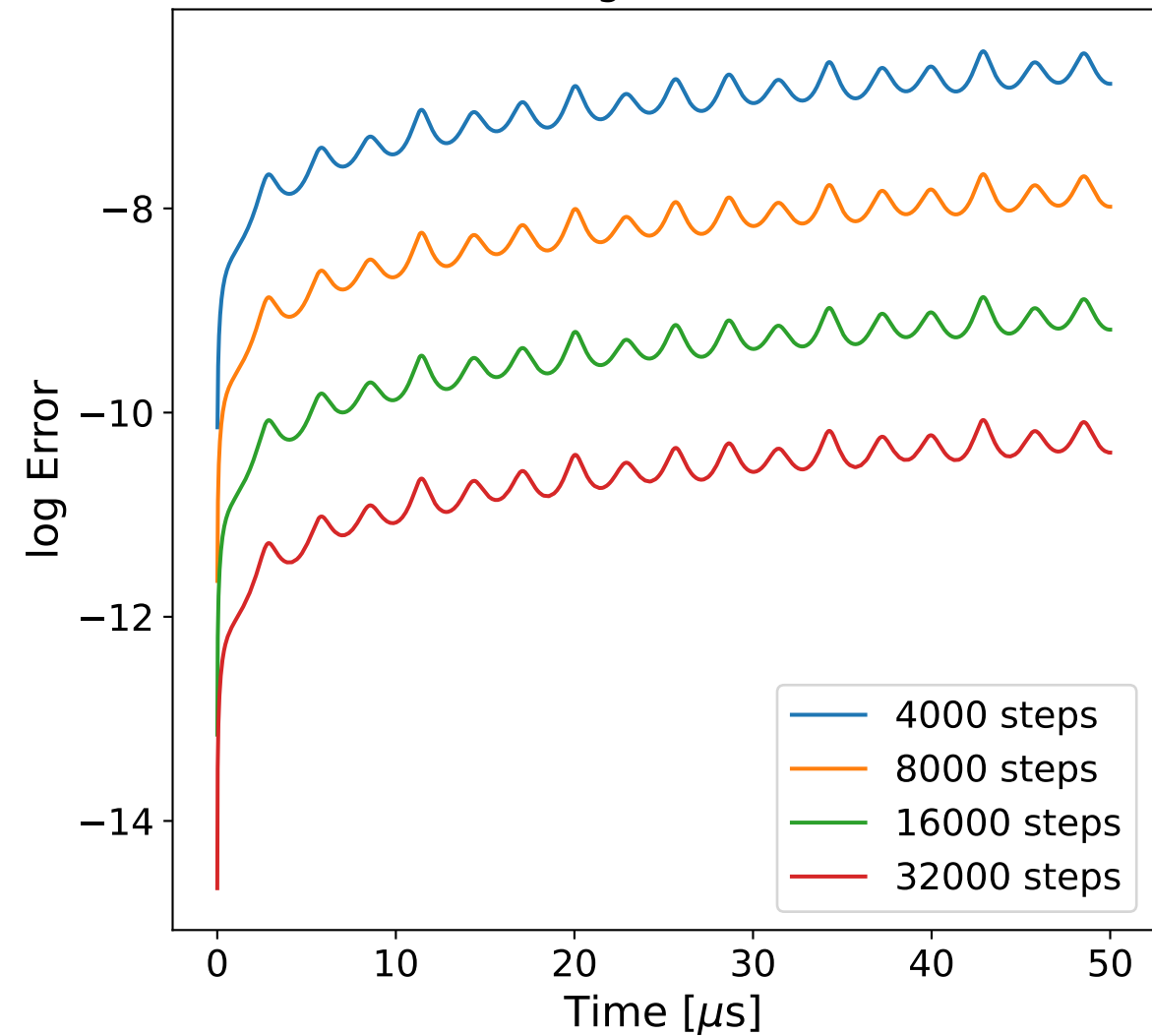
Runge Kutta 4
