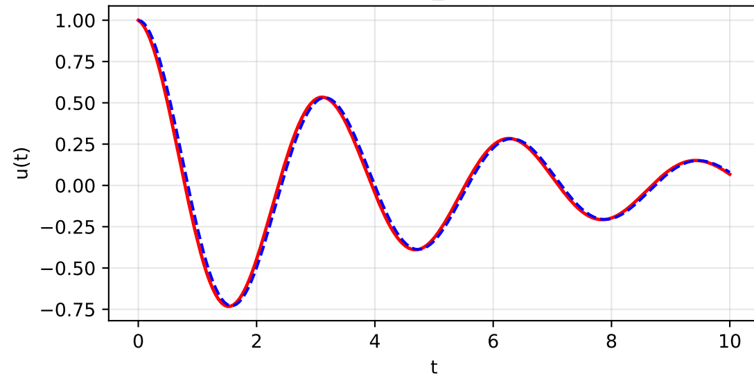
KANN_cheb
