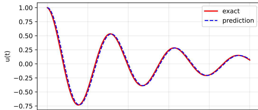
MLP
