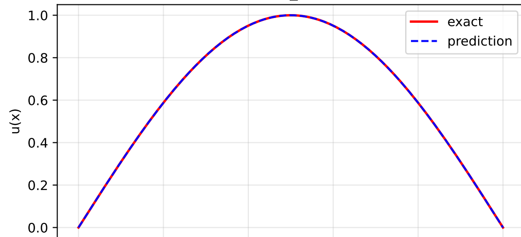
KANN_cheb
