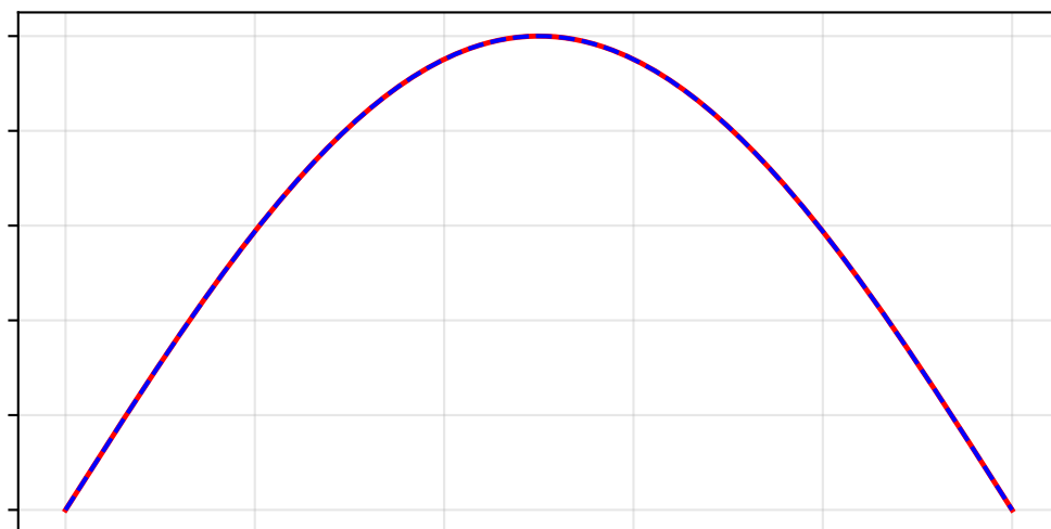
MLP
