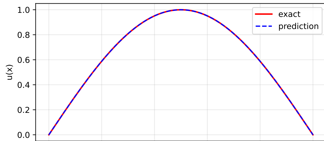
MLP
