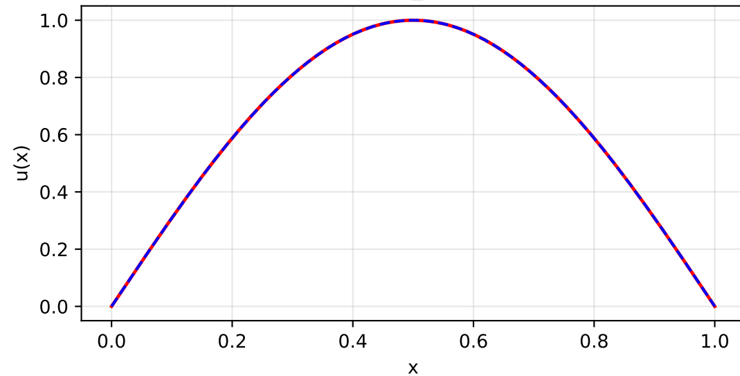
KANN_cheb
