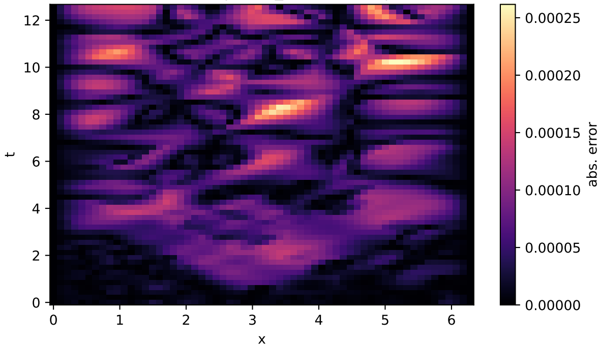
1D Wave - |KANN_cheb - exact|
