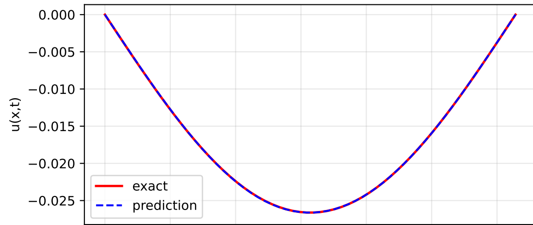
MLP
