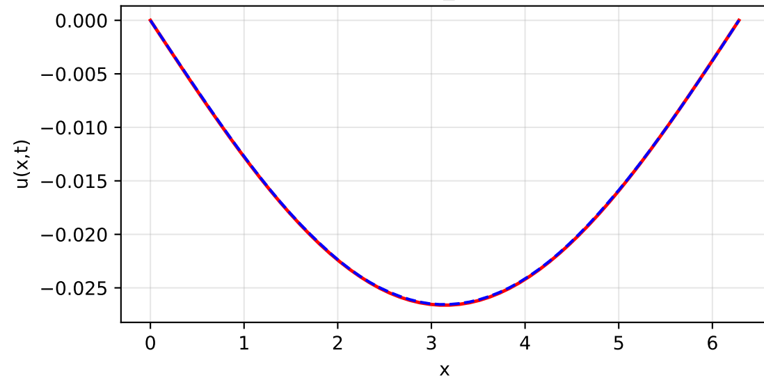
KANN_cheb
