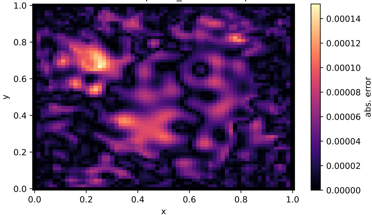
2D Poisson - |KANN_cheb - exact|
