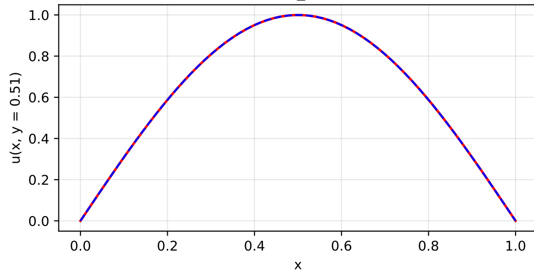
KANN_cheb
