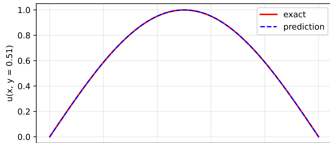
MLP
