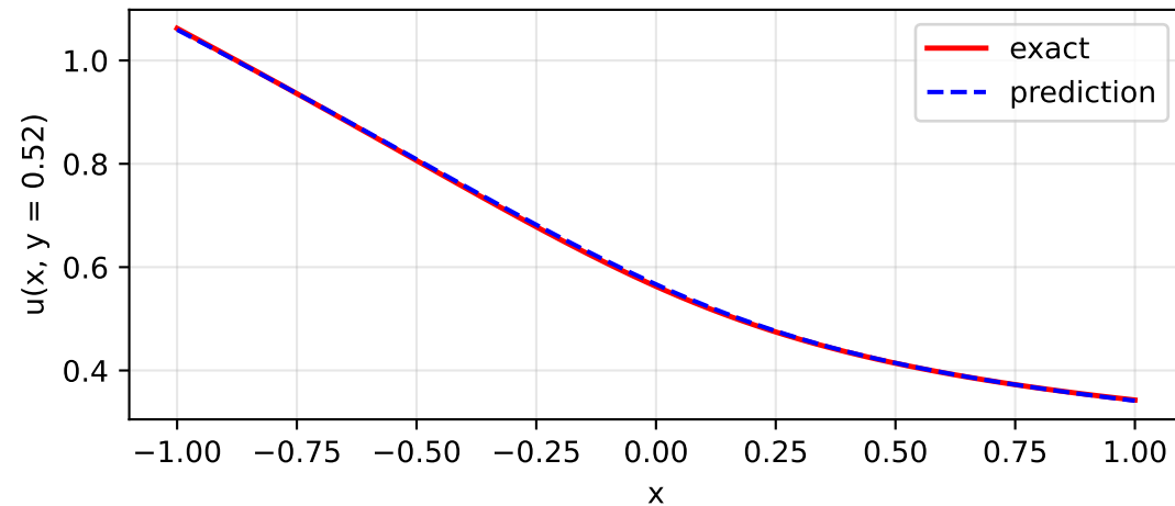
MLP
