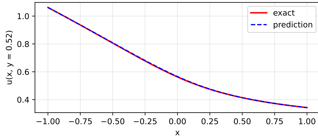
MLP
